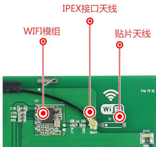
图 1-4 WIFI 配置图
