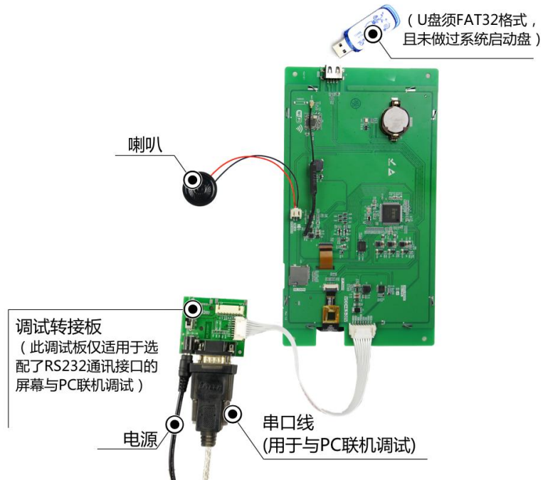
图 1-5 调试工具图
