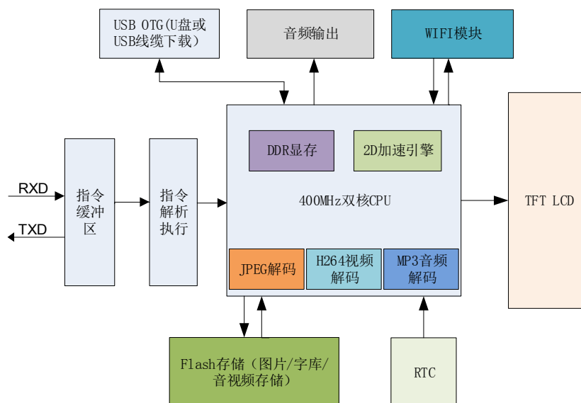
图 10-1 物联型串口屏内部结构图
