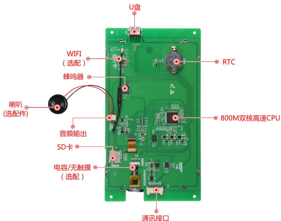
图 1-3 硬件配置图
