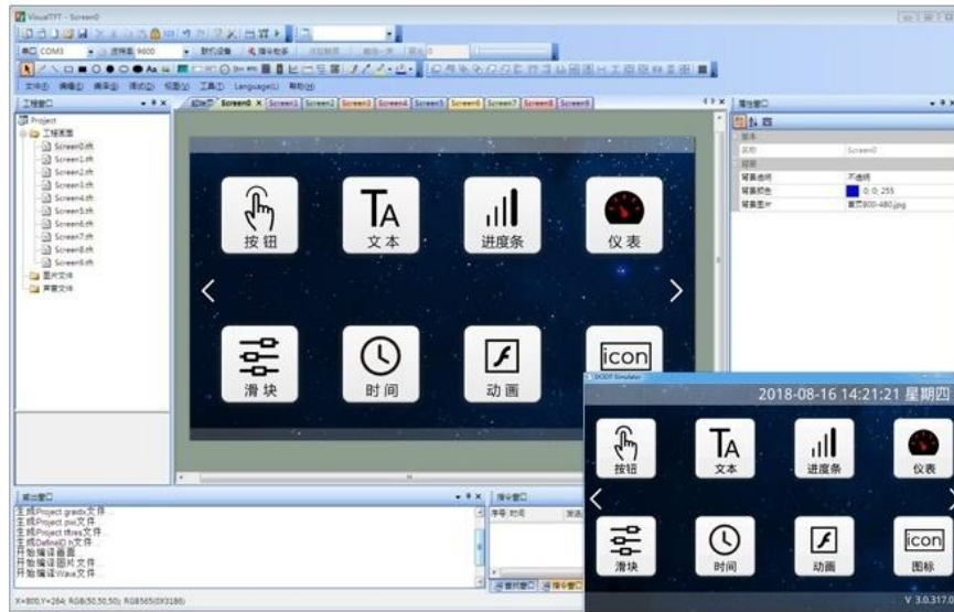
图 11-1 VisualTFT 主界面
