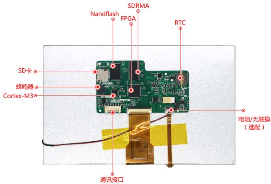
图 1-3 硬件配置图
