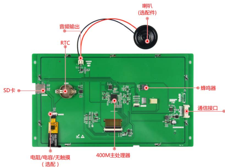
图 1-4 硬件配置图
