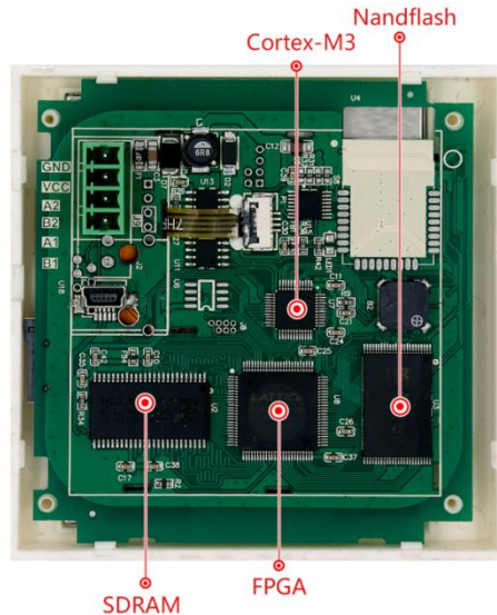
1-1 硬件配置图
