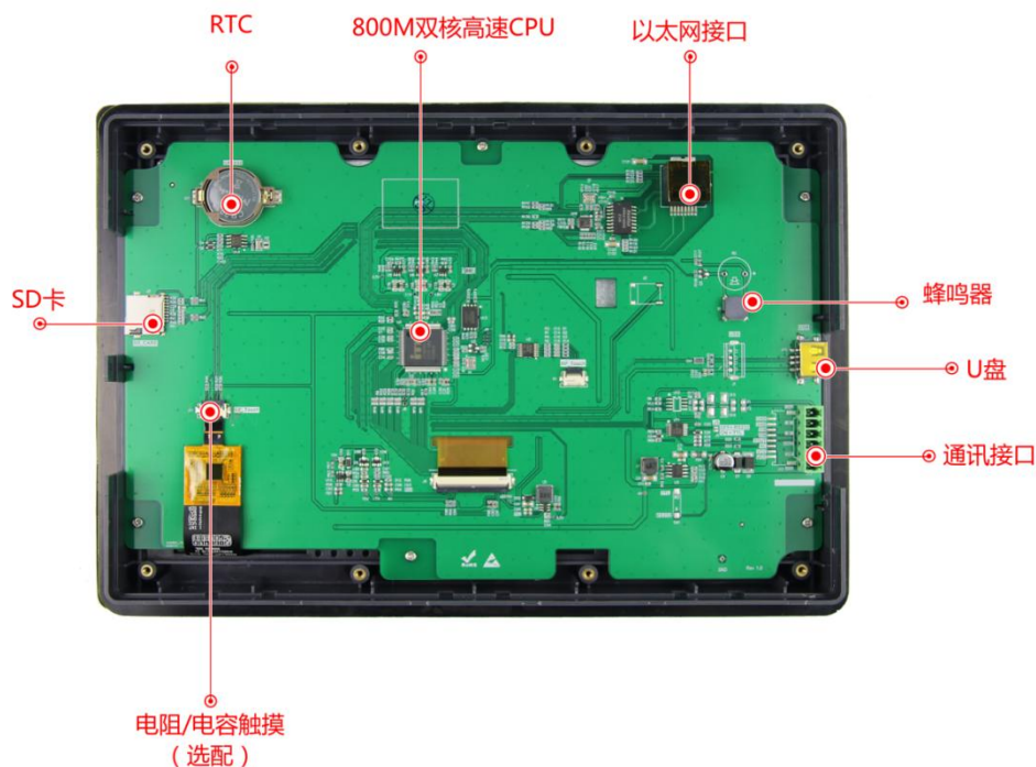
图 1-3 硬件配置图
