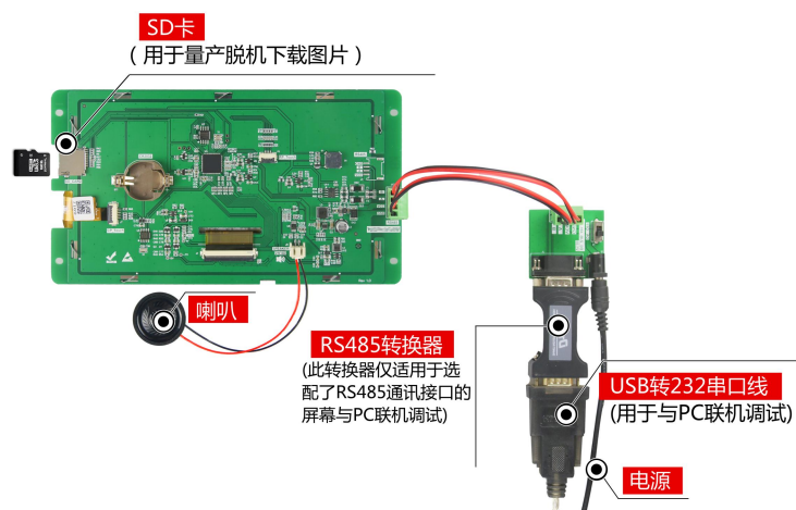
图 1-5 调试工具图
