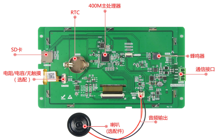
图 1-4 硬件配置图
