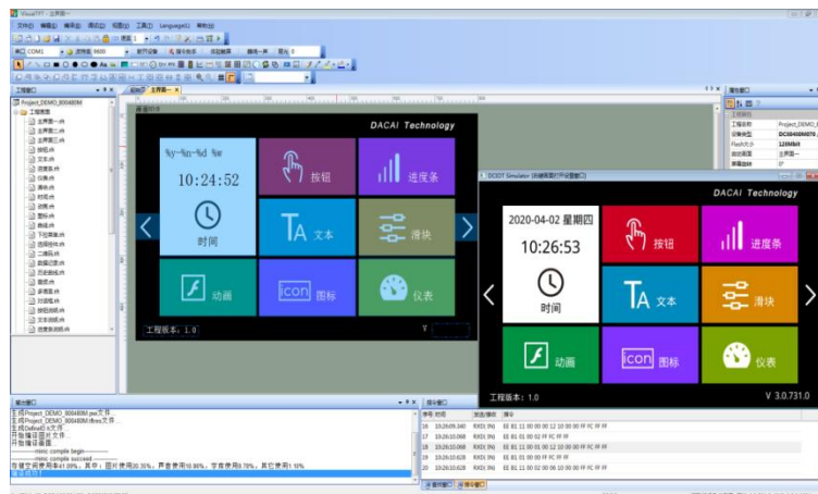
图 10-1 VisualTFT 主界面
