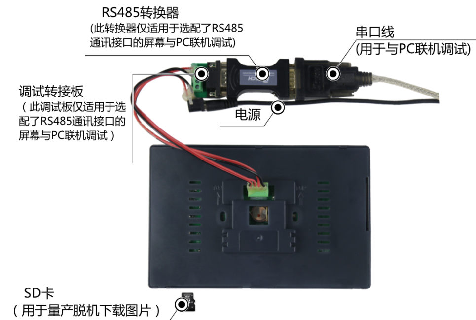
图 1-4 调试工具图
