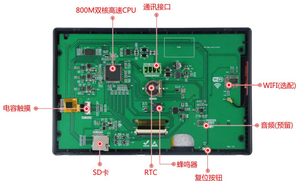
图 1-2 硬件配置图
