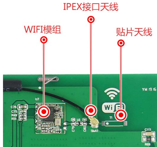
图 1-3 WIFI 配置图
