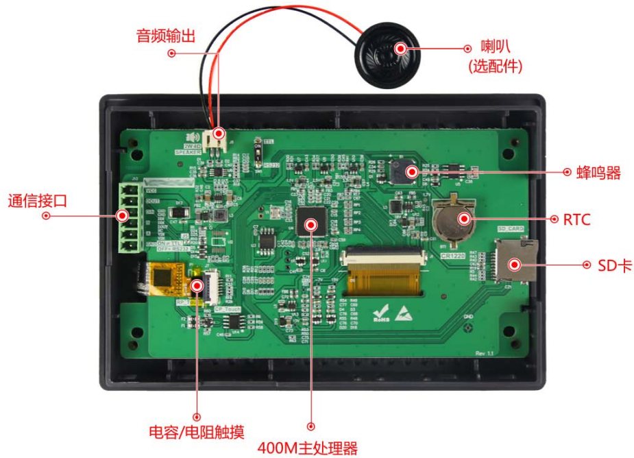
图 1-3 硬件配置图
