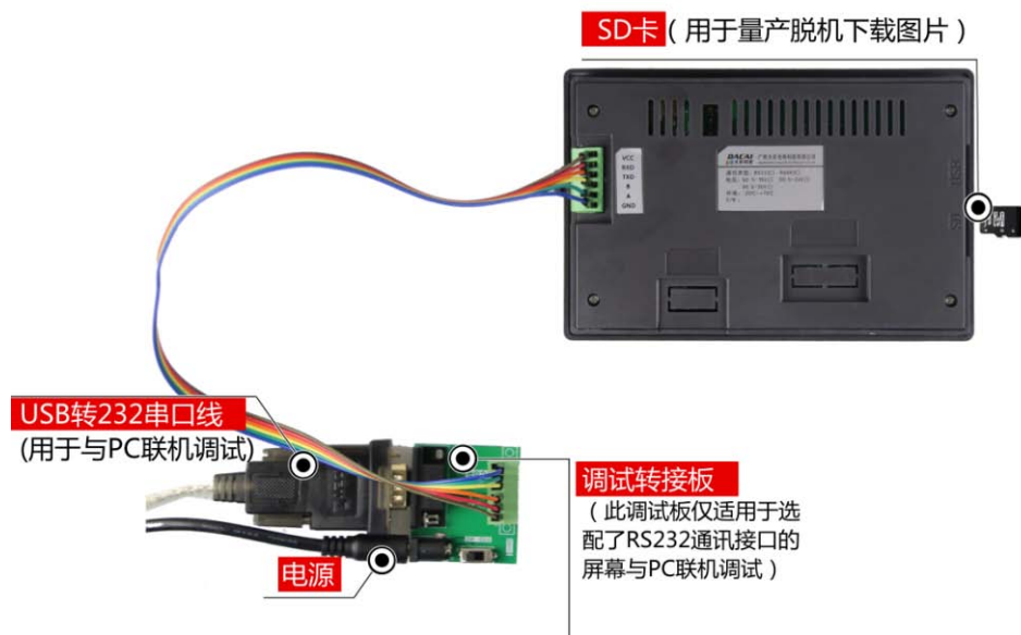
图 1-4 RS232 调试工具图
