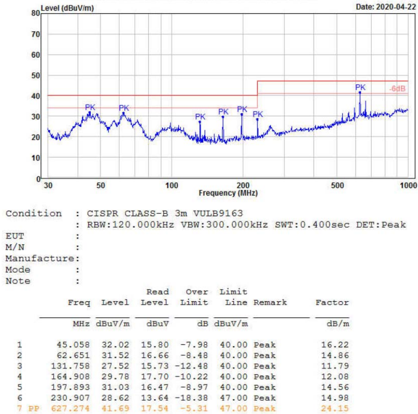
图 6-7 辐射测试垂直方向
