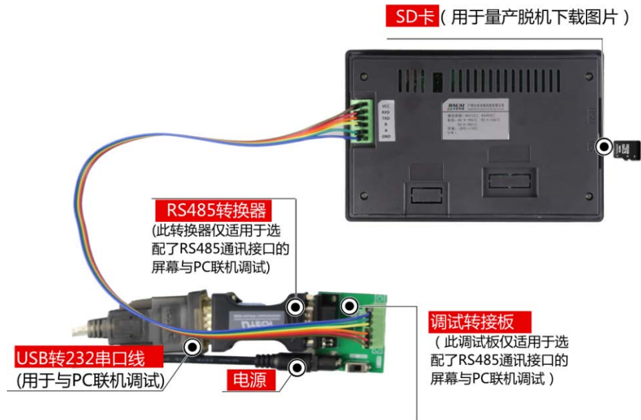
图 1-5 RS485 调试工具图
