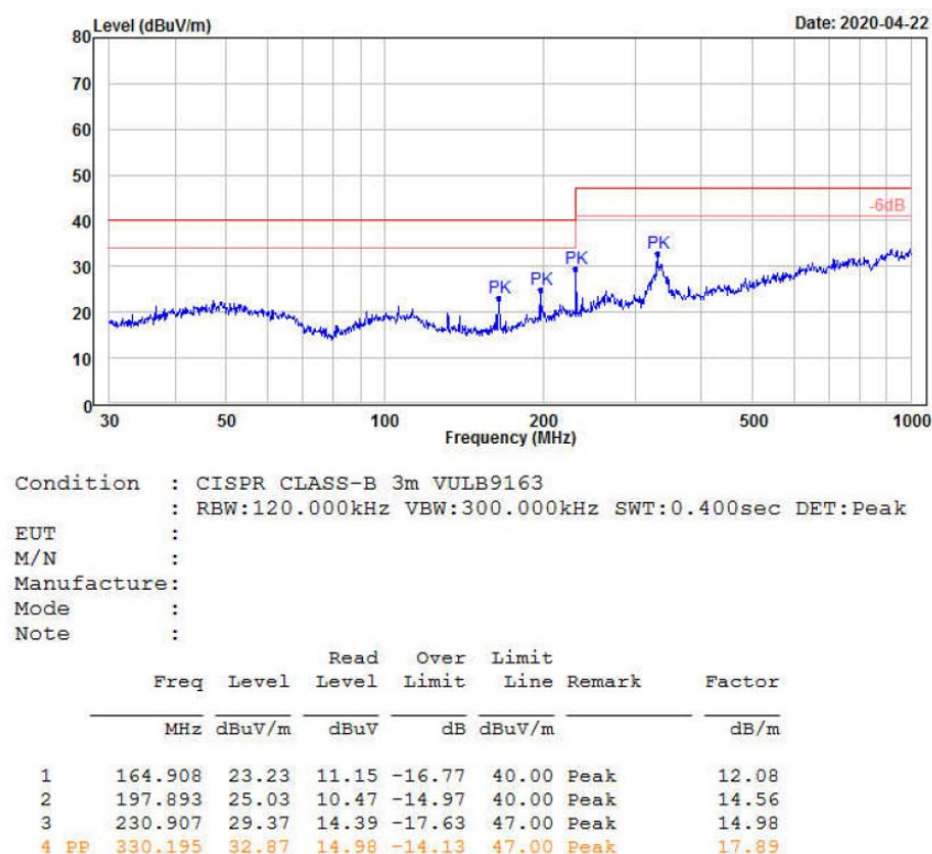
图 6-6 辐射测试水平方向
