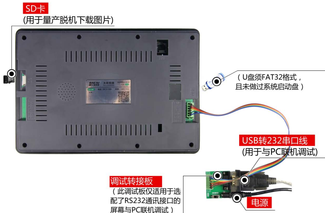
图 1-4 RS232 调试工具
