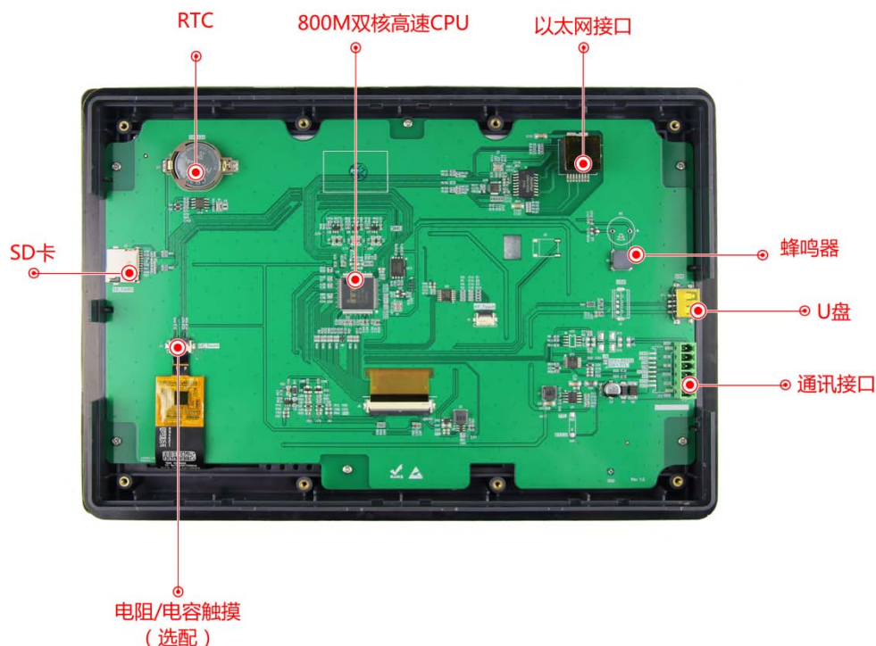
图 1-3 硬件配置图
