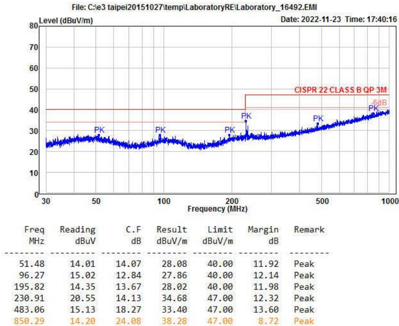
图 5-6 辐射测试水平方向
