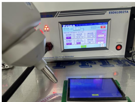
图 5-2 ESD 测试图
