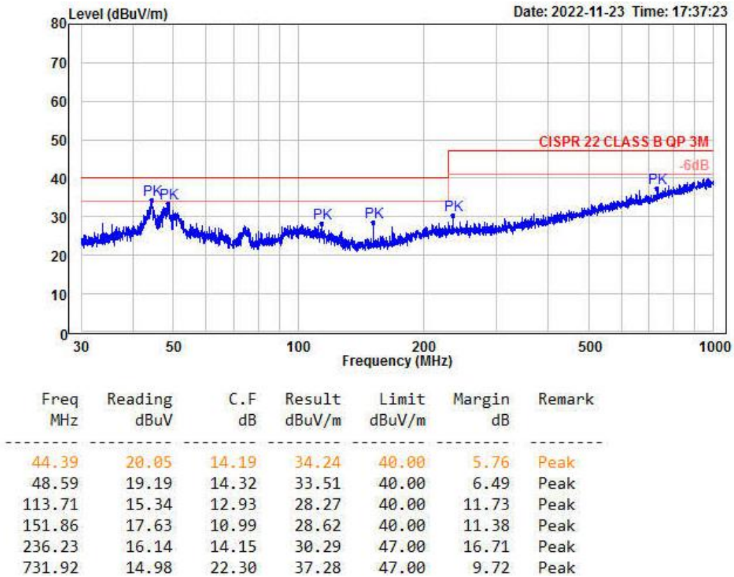
图 5-7 辐射测试垂直方向
