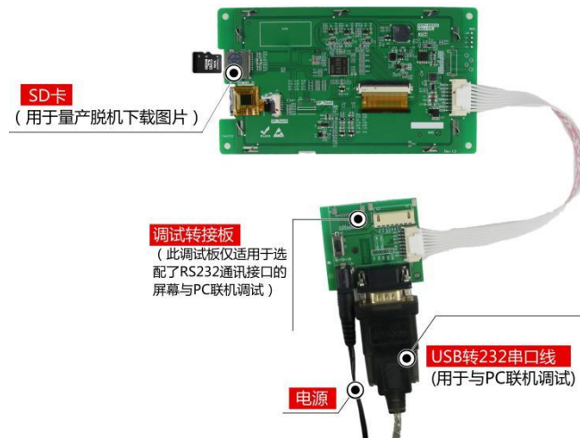
图 1-5 调试工具图
