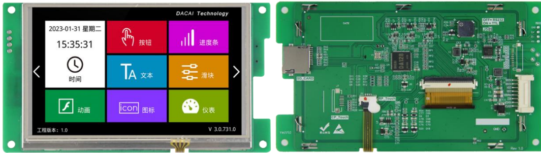
图 1-1 5.0 寸电阻触摸参考图
