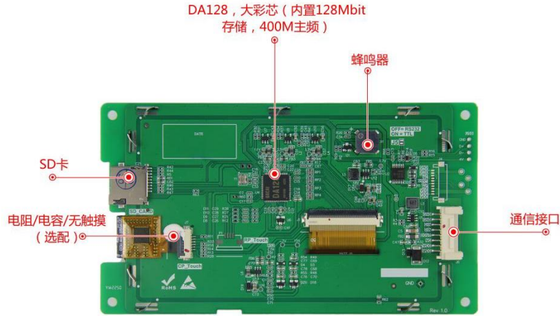
图 1-4 硬件配置图
