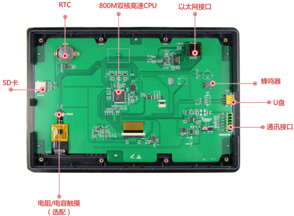
图 1-3 硬件配置图
