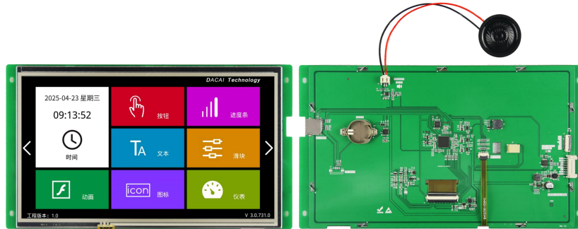
图 1-1 10.1 寸电阻触摸参考图
