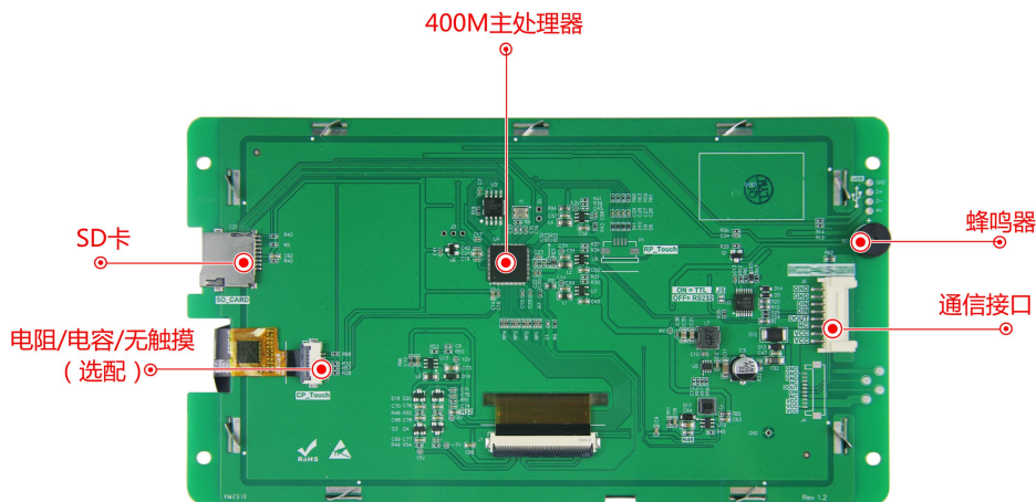
图 1-4 硬件配置图
