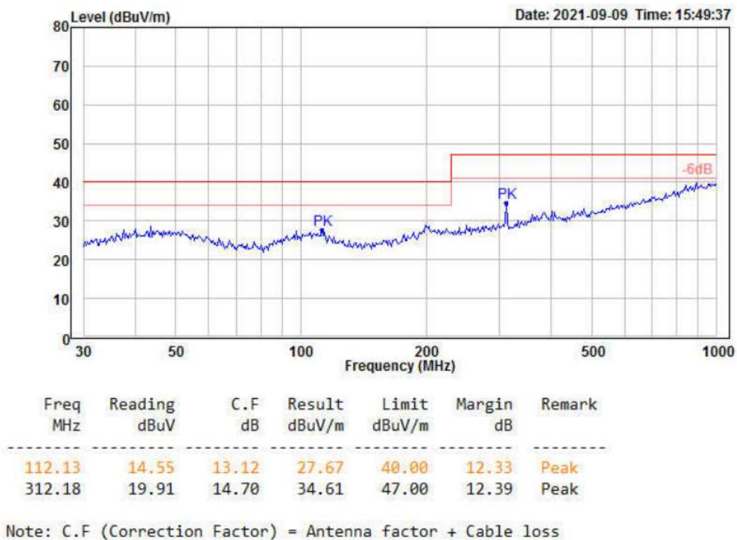
图 4-5 RE 测试水平方向
