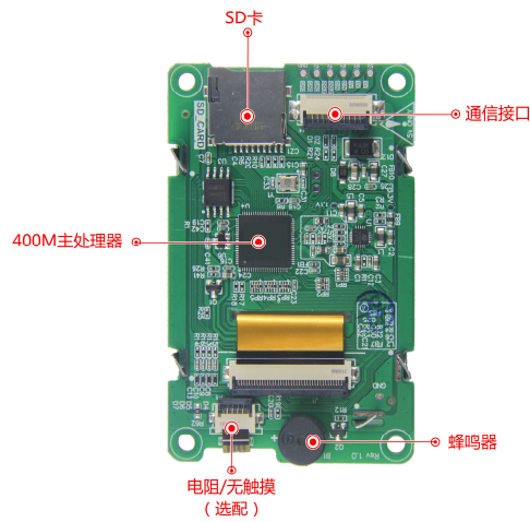
图 1-3 硬件配置图
