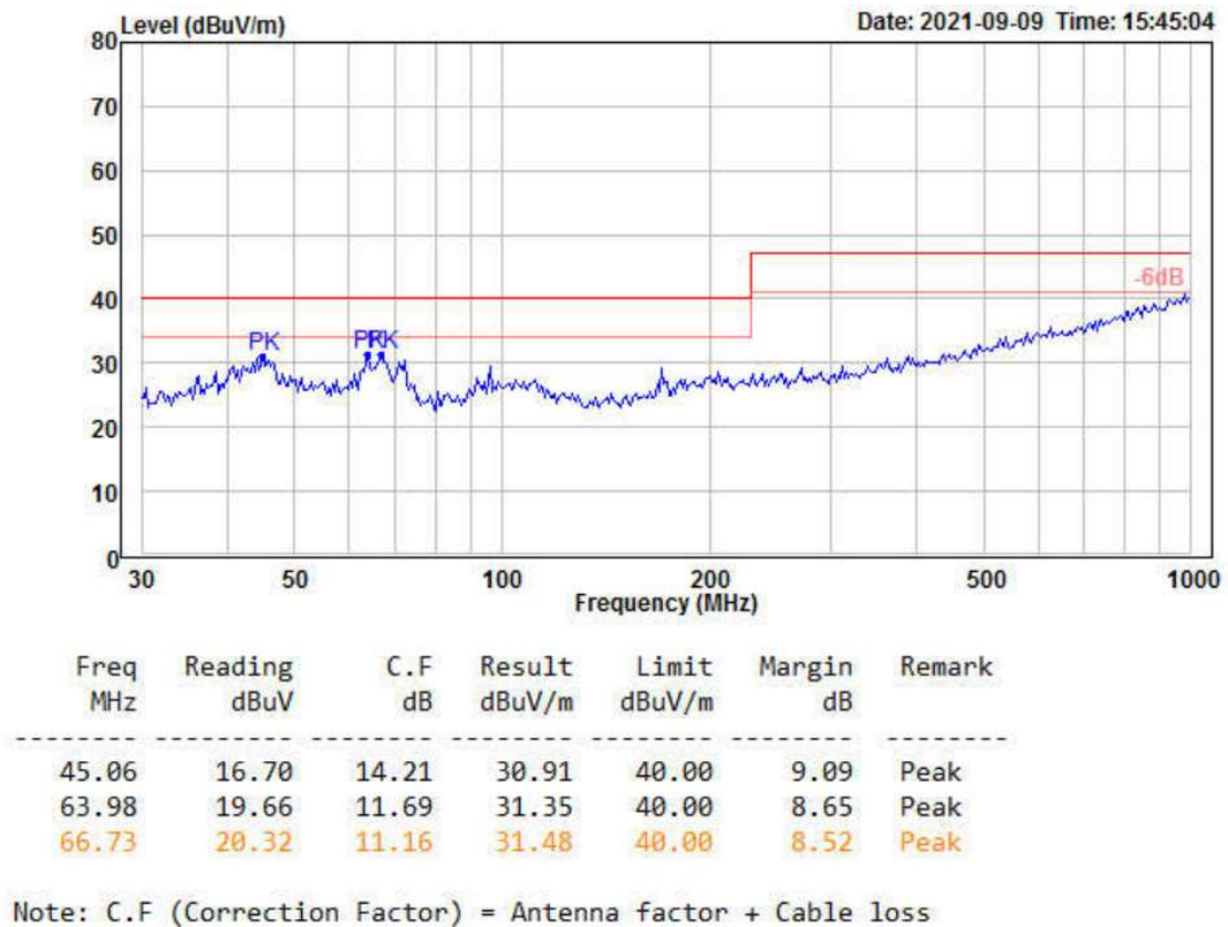
图 4-6 RE 测试垂直方向
