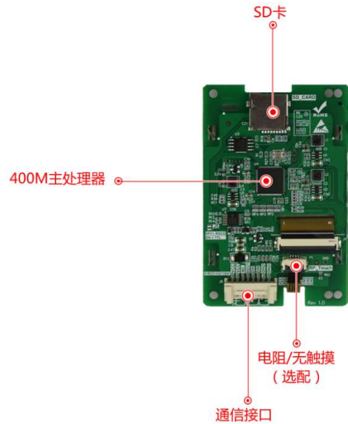
图 1-3 硬件配置图
