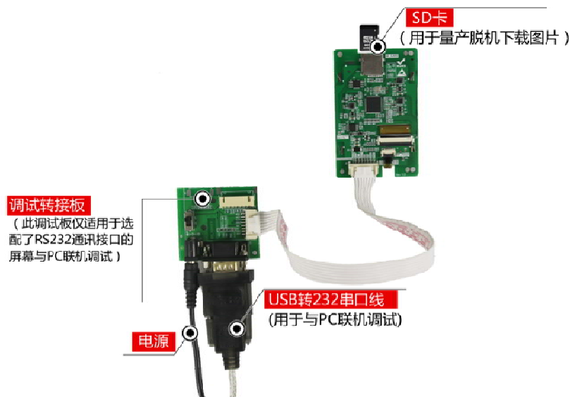
图 1-4 调试工具图
