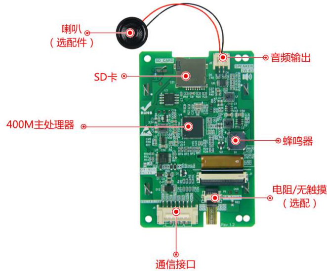
图 1-3 硬件配置图
