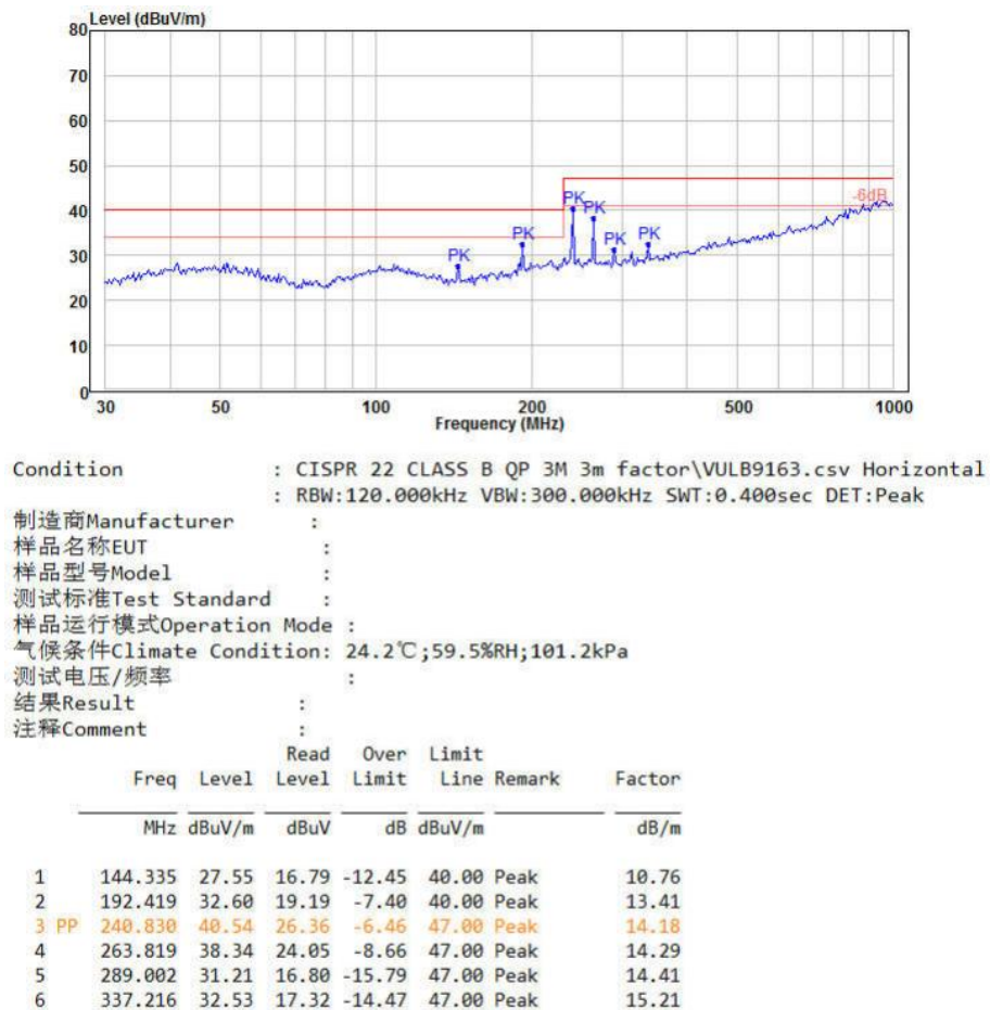
图 4-5 RE 测试水平方向
