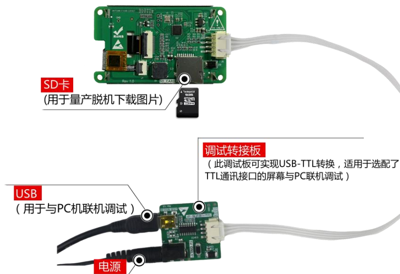
图 1-3 调试工具图
