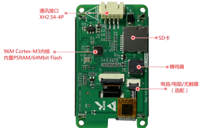
图 1-2 硬件配置图
