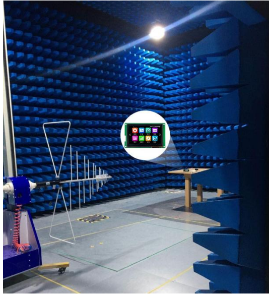
图 4-4 RE 测试图
