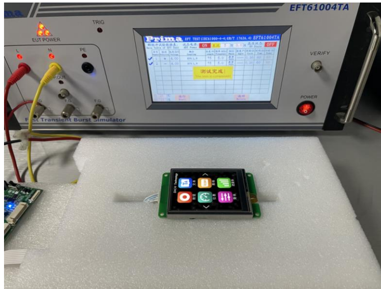
图 4-3 EFT 测试图
