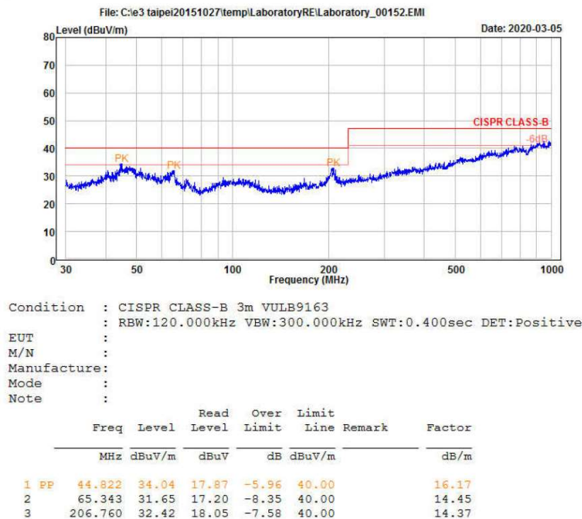
图 4-6 RE 测试垂直方向
