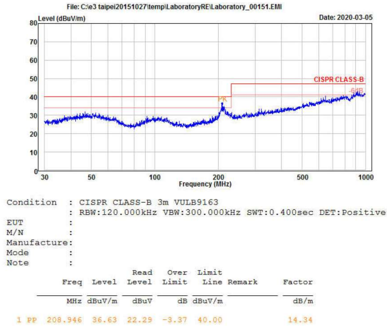
图 4-5 RE 测试水平方向
