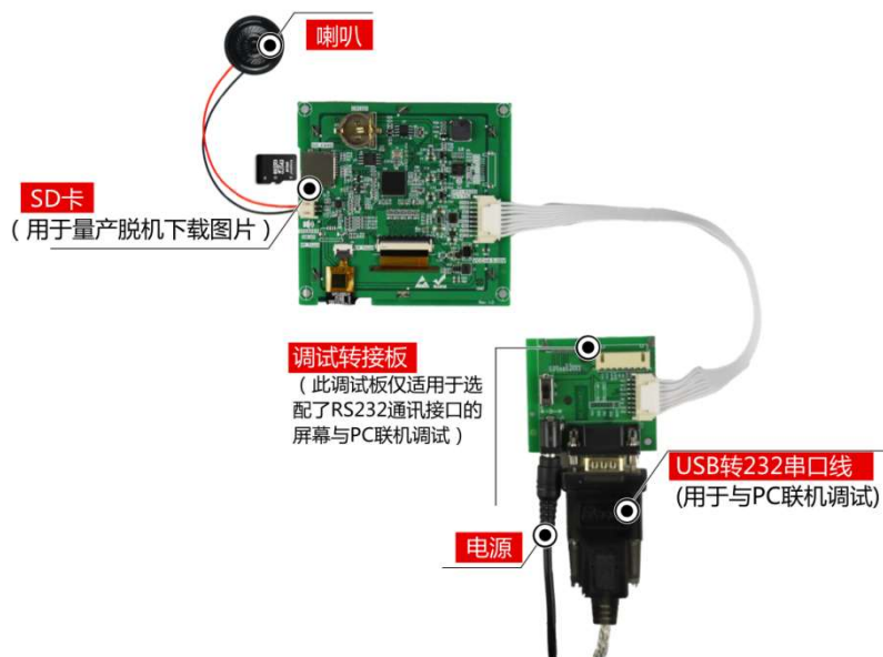
图 1-5 调试工具图
