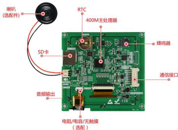
图 1-4 硬件配置图
