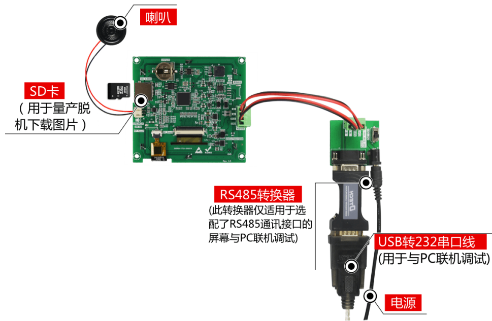
图 1-5 调试工具图
