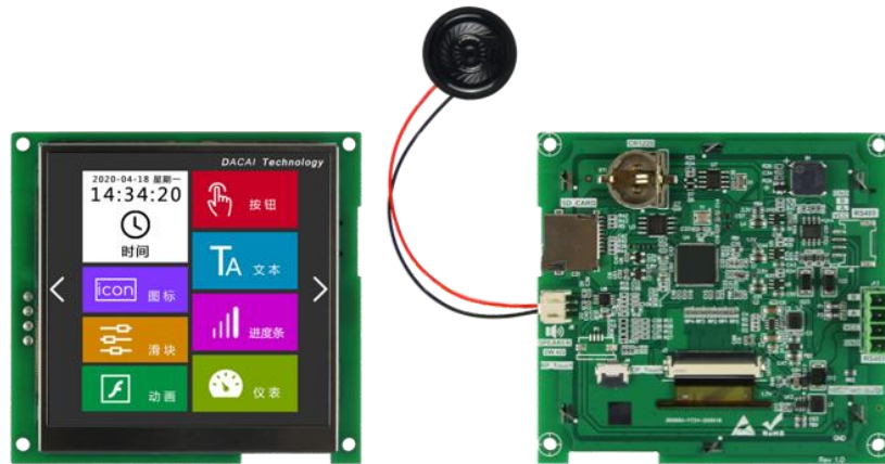
图 1-3 4.0 寸无触摸参考图
