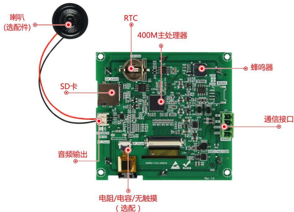
图 1-4 硬件配置图
