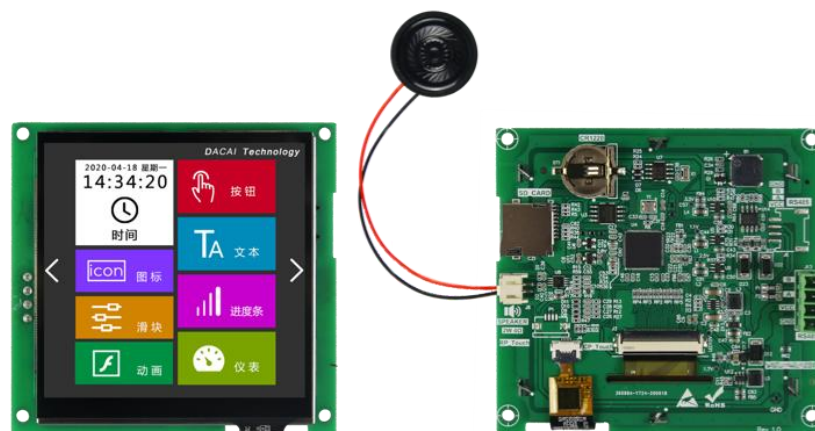
图 1-2 4.0 寸电容触摸参考图
