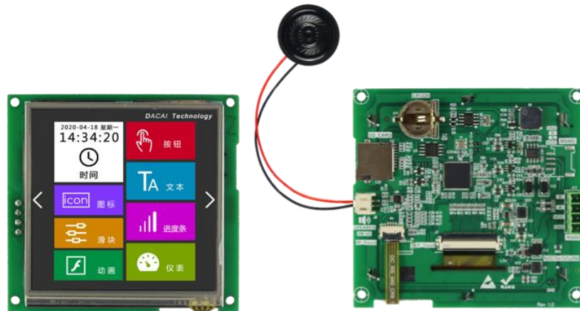
图 1-1 4.0 寸电阻触摸参考图
