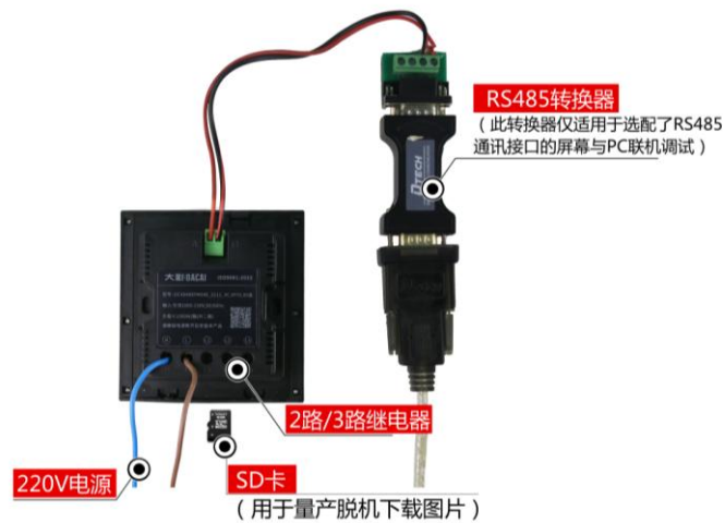
图 1-6 调试工具图
