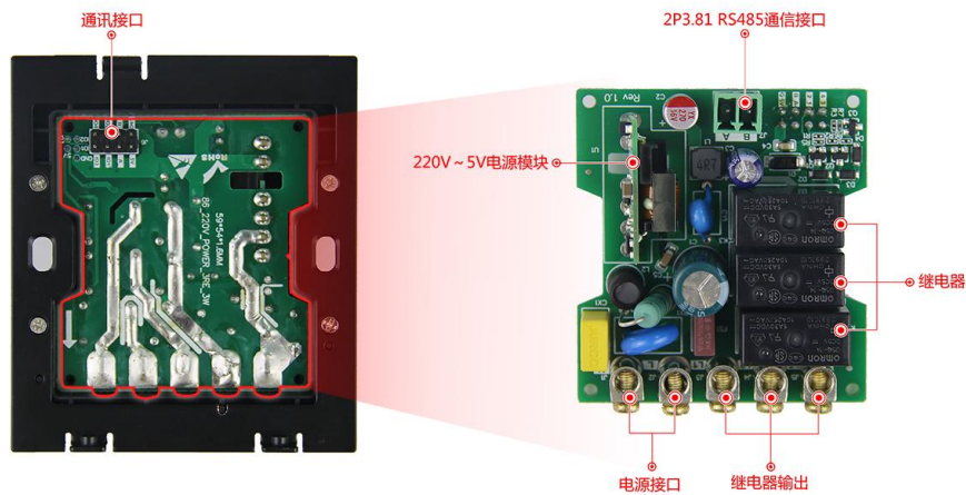
图 1-5 电源板硬件配置图
