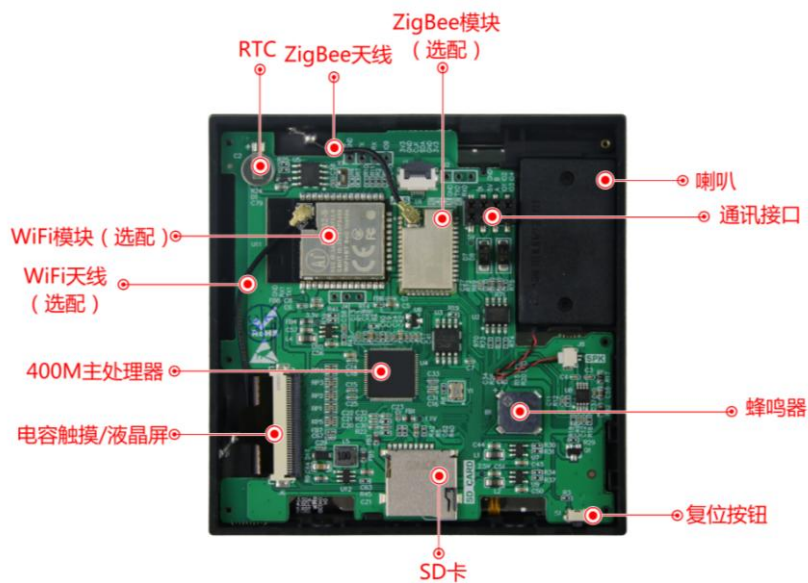
图 1-3 带 WiFi、ZigBee 硬件配置图
