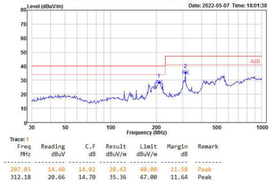
图 5-5 RE 测试水平方向
