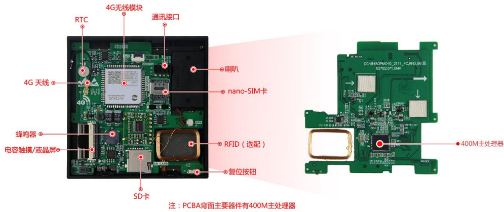
图 1-4 带 4G、RFID 硬件配置图
