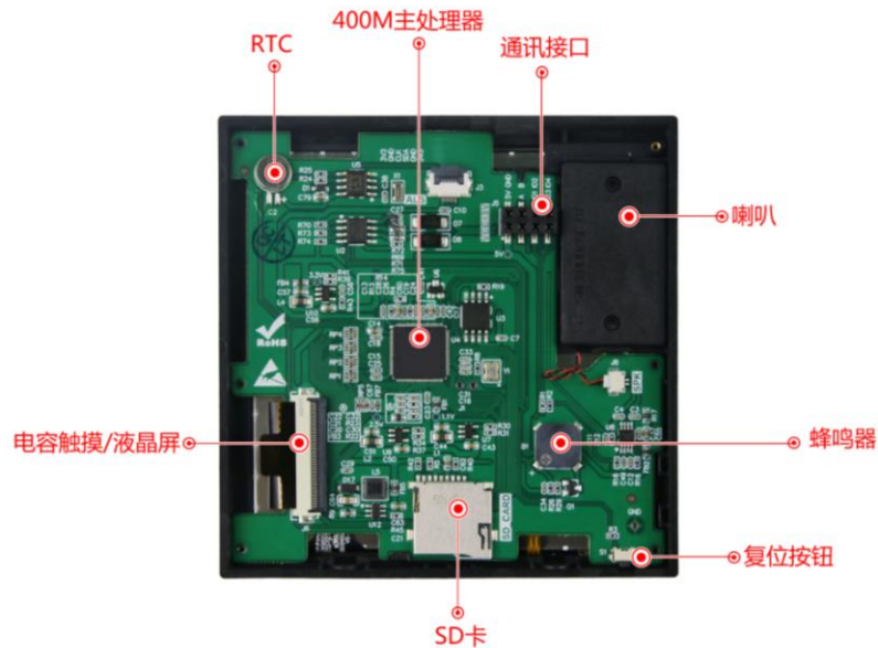
图 1-2 基础版硬件配置图
