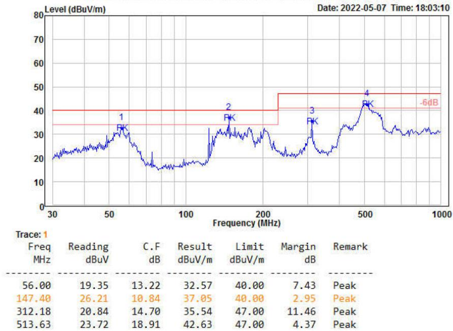
图 5-6 RE 测试垂直方向
