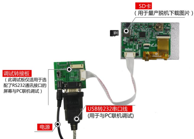
图 1-5 调试工具图
