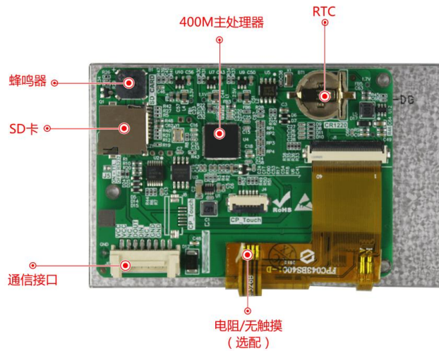
图 1-4 硬件配置图
