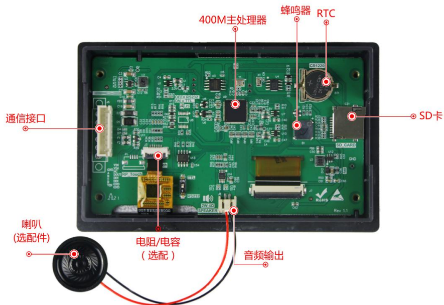
图 1-3 硬件配置图
