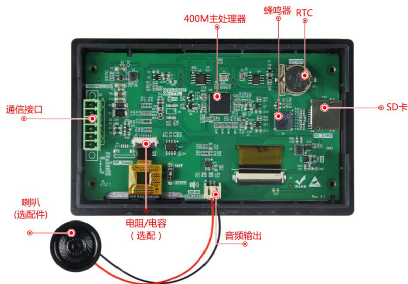
图 1-3 硬件配置图
