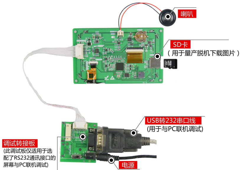
图 1-5 调试工具图
