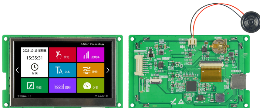
图 1-3 4.3 寸无触摸参考图
