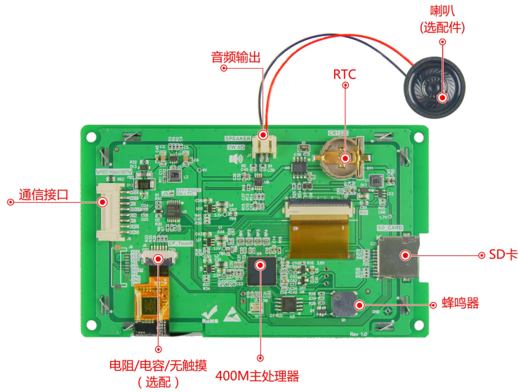
图 1-4 硬件配置图
