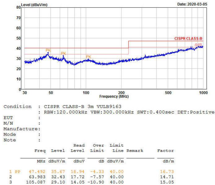
图 4-6 RE 测试垂直方向
