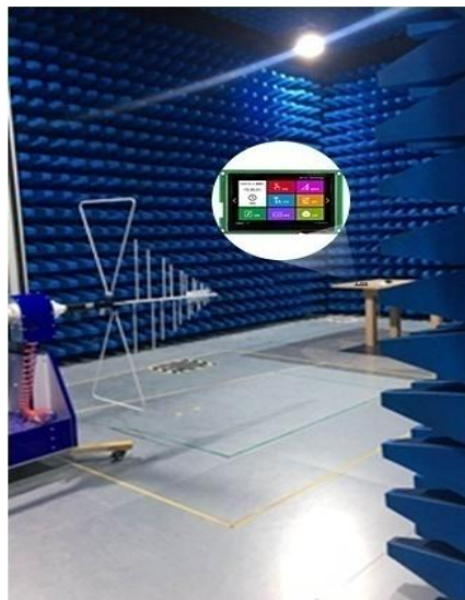
图 4-4 RE 测试图
