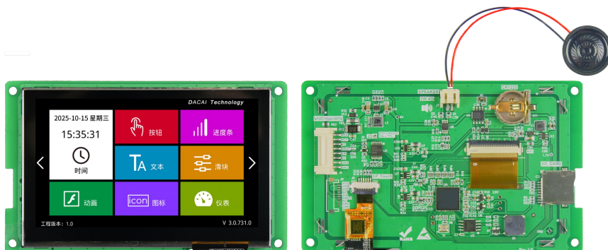
图 1-2 4.3 寸电容触摸参考图
