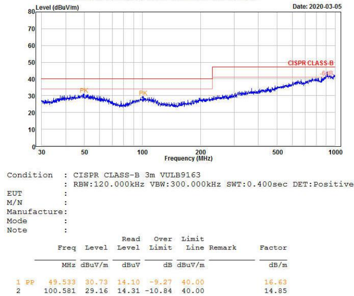
图 4-5 RE 测试水平方向
