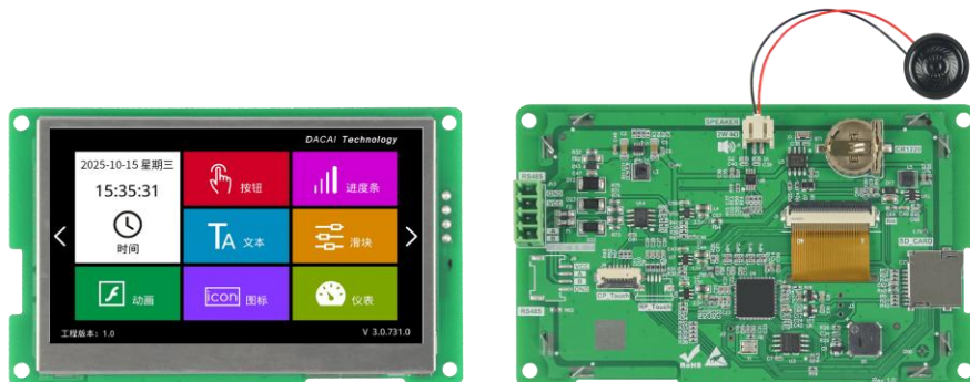
图 1-3 4.3 寸无触摸参考图
