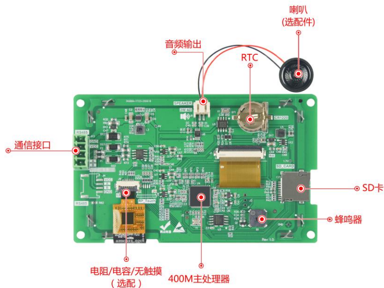
图 1-4 硬件配置图
