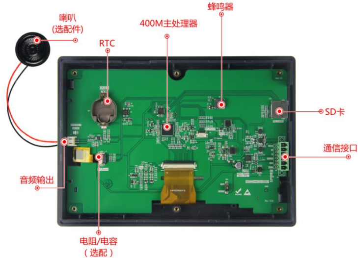
图 1-3 硬件配置图
