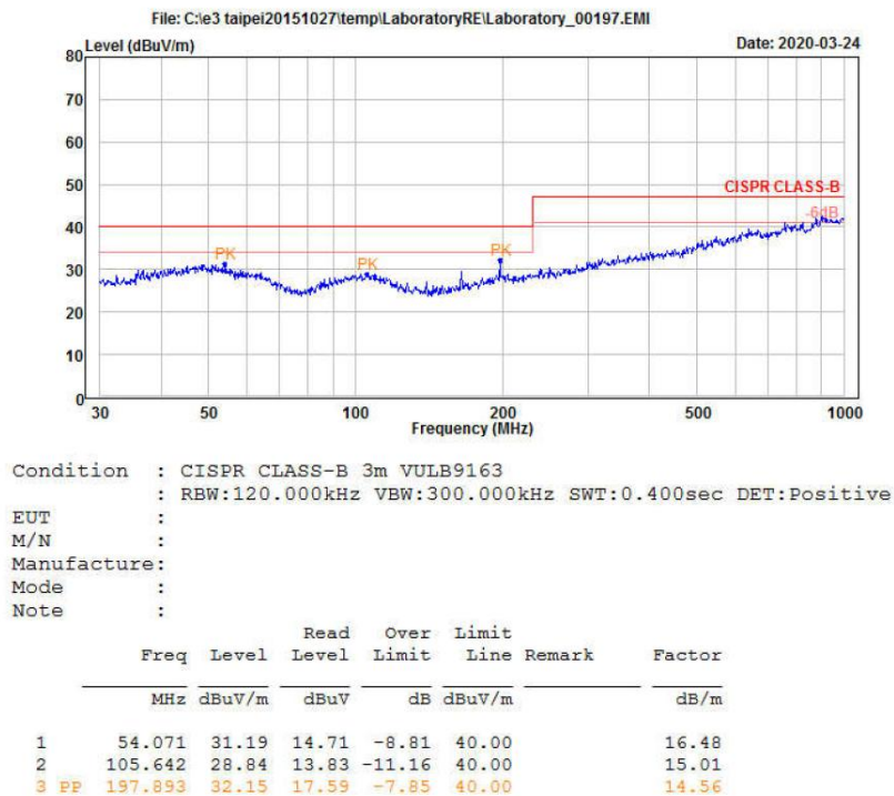
图 5-5 RE 测试水平方向
