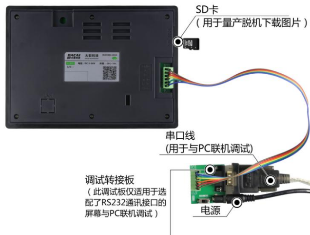
图 1-4 RS232 调试工具图
