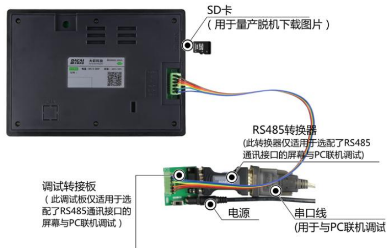
图 1-5 RS485 调试工具图
