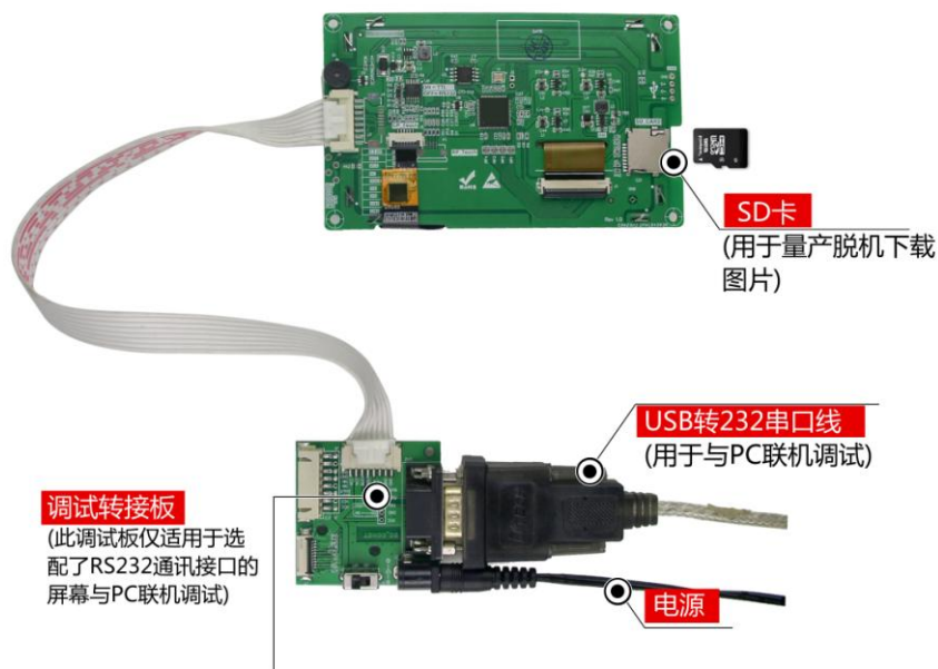
图 1-5 调试工具图
