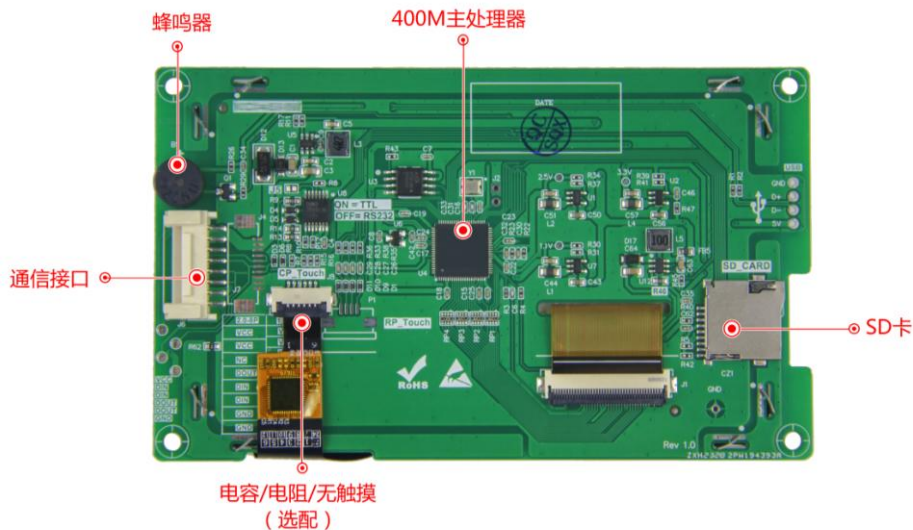
图 1-4 硬件配置图
