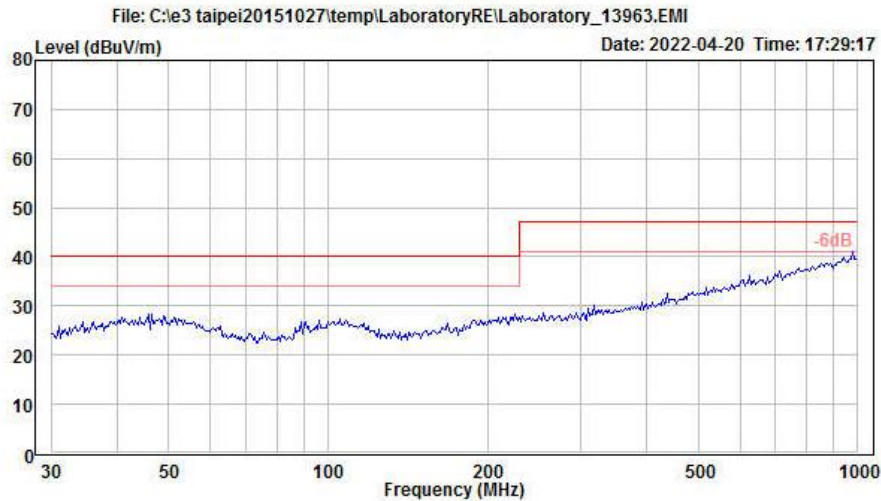
图 4-5 RE 测试水平方向
