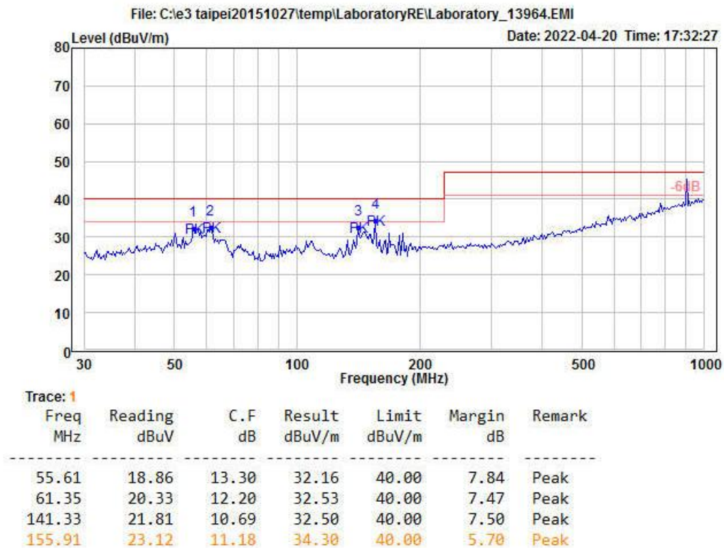
图 4-6 RE 测试垂直方向
