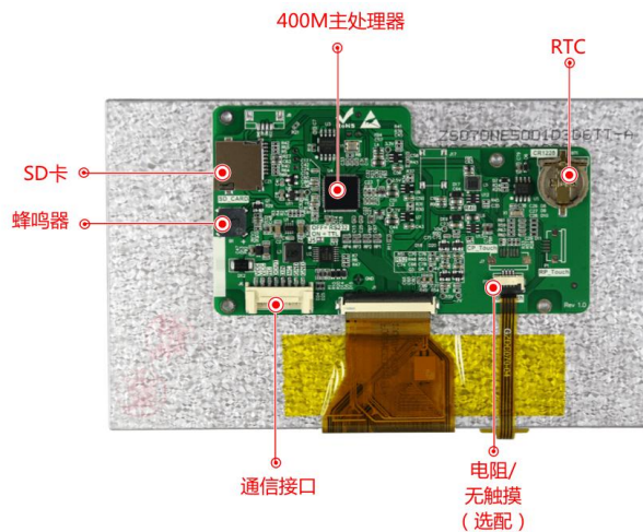
图 1-3 硬件配置图
