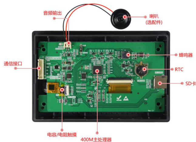
图 1-3 硬件配置图
