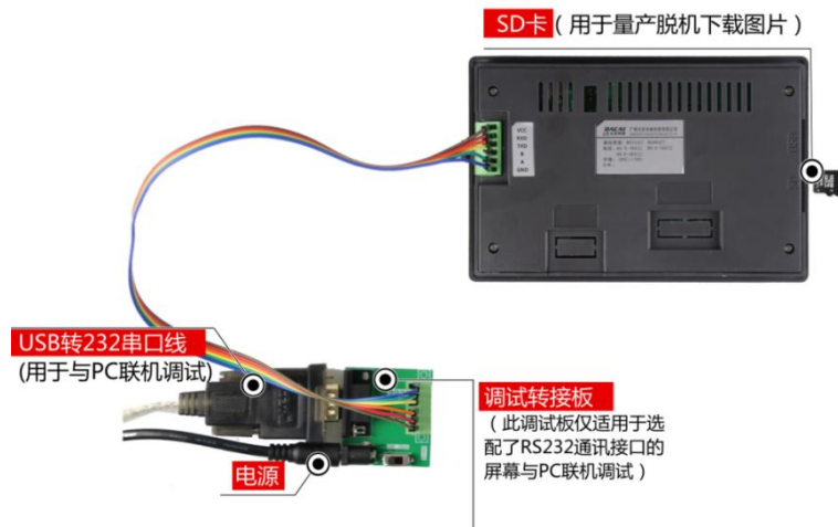
图 1-4 RS232 调试工具图
