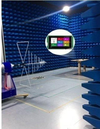
图 5-4 RE 测试图
