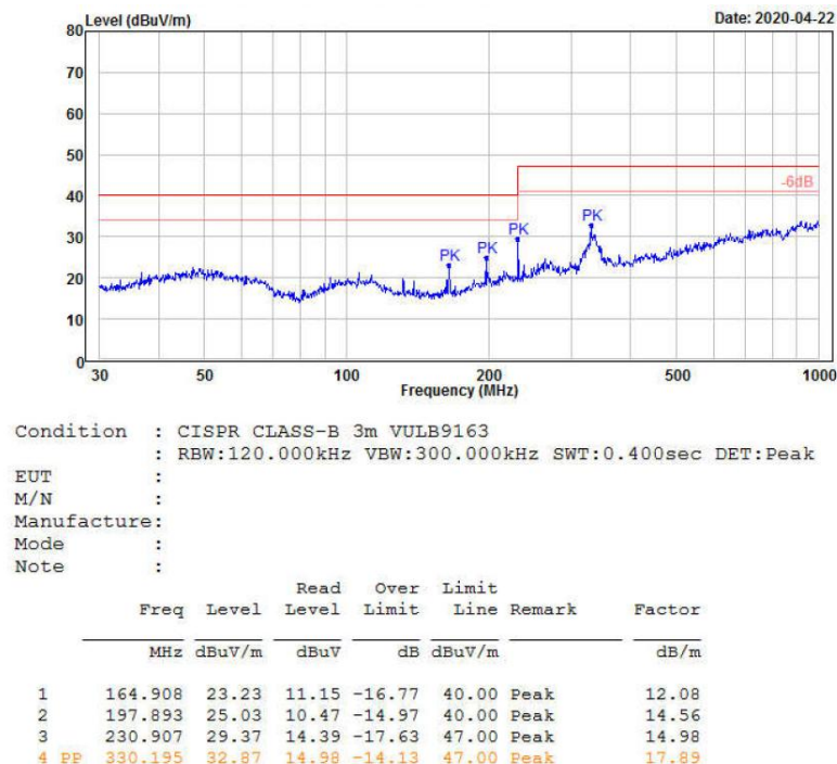
图 5-5 RE 测试水平方向
