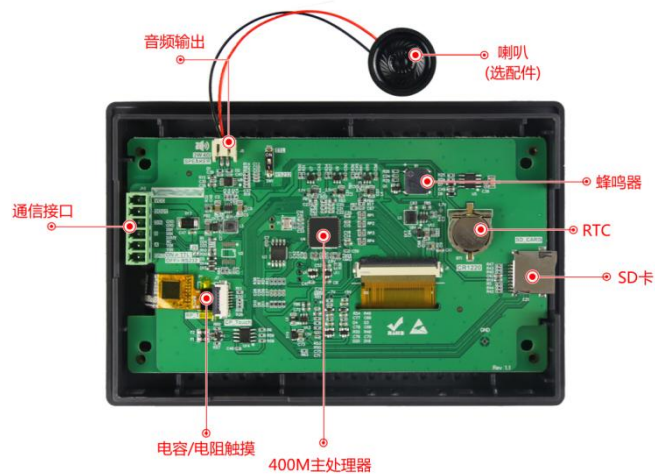
图 1-3 硬件配置图
