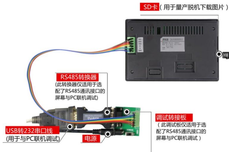
图 1-5 RS485 调试工具图
