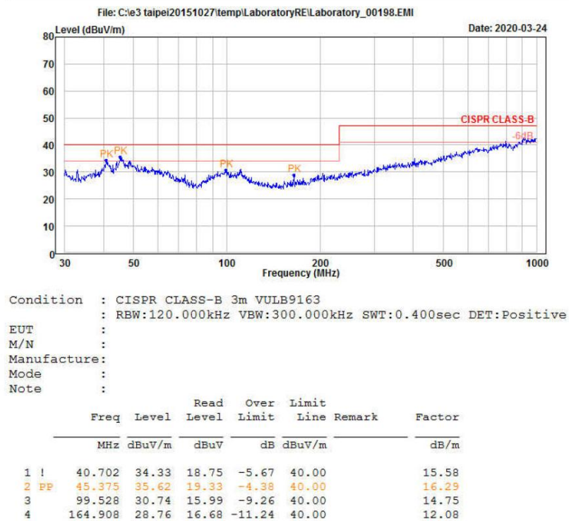
图 5-6 RE 测试垂直方向
