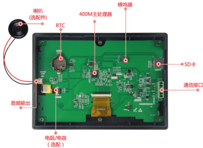
图 1-3 硬件配置图
