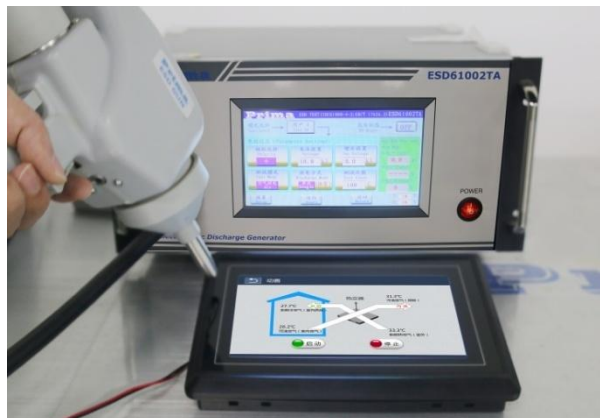
图 5-2 ESD 测试图
