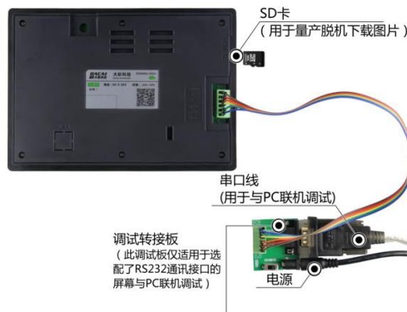
图 1-4 RS232 调试工具图
