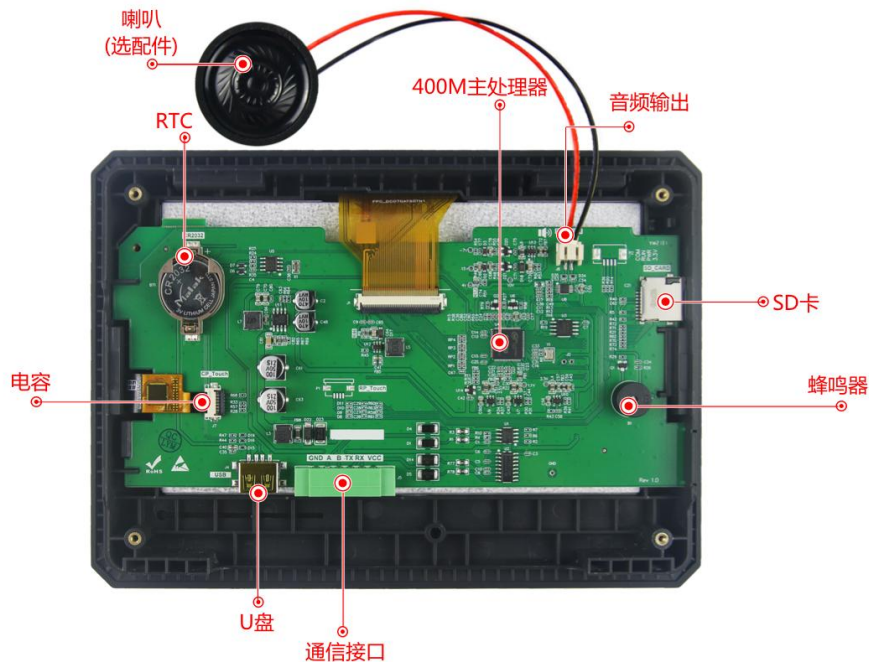
图 1-2 硬件配置图
