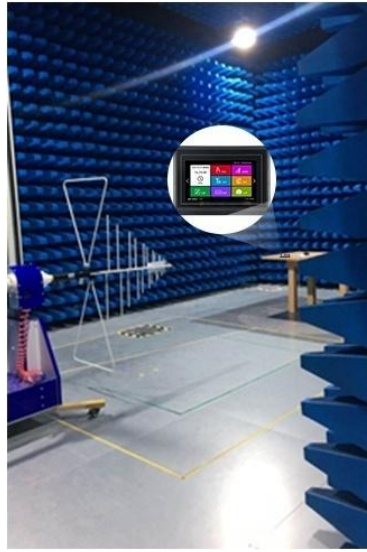
图 5-4 RE 测试图
