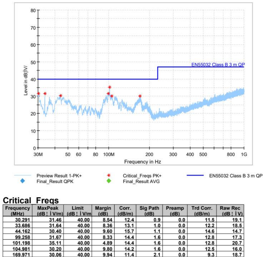
图 5-6 RE 测试垂直方向
