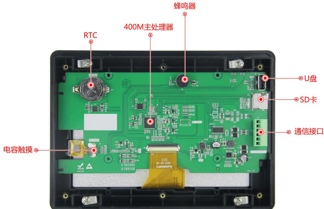
图 1-2 硬件配置图
