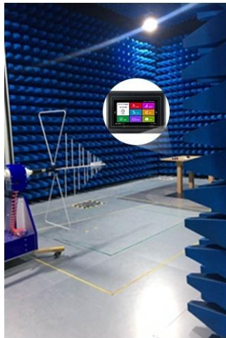
图 5-4 RE 测试图
