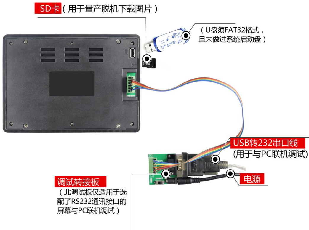
图 1-3 RS232 调试工具图
