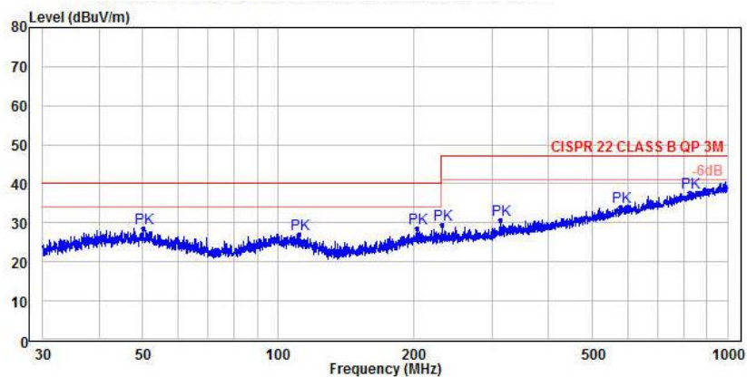
图 5-5 RE 测试水平方向
