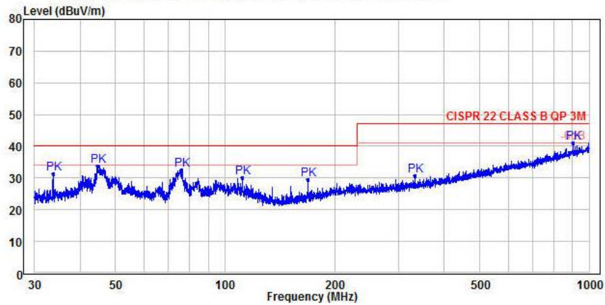
图 5-6 RE 测试垂直方向
