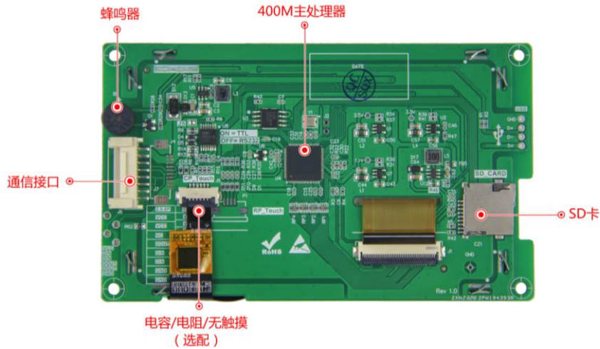
图 1-4 硬件配置图
