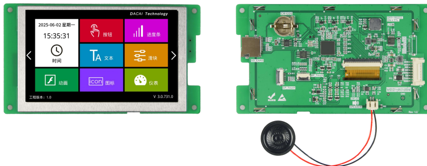
图 1-3 5.0 寸无触摸参考图
