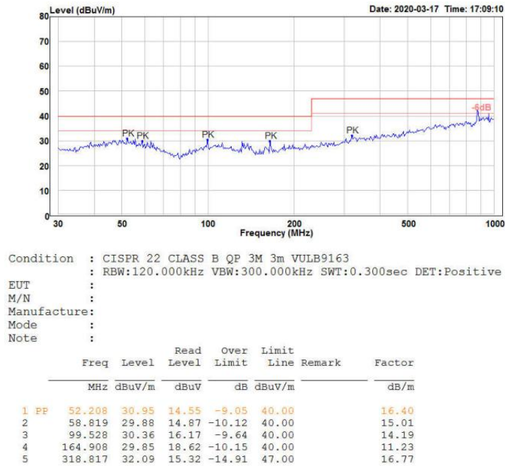
图 4-5 RE 测试水平方向
