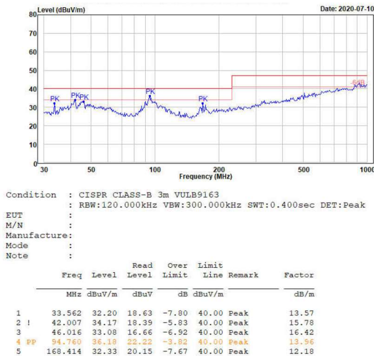
图 4-6 RE 测试垂直方向
