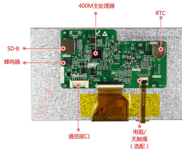
图 1-3 硬件配置图
