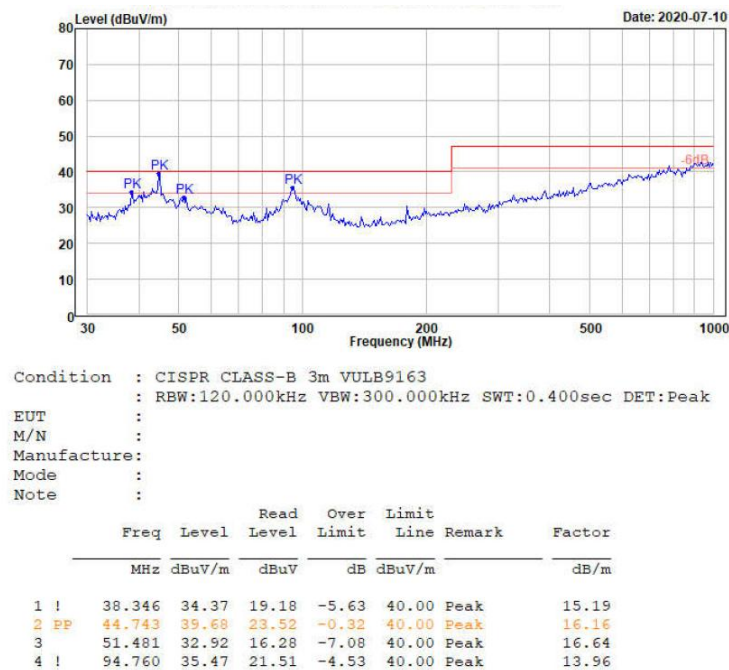
图 4-6 RE 测试垂直方向
