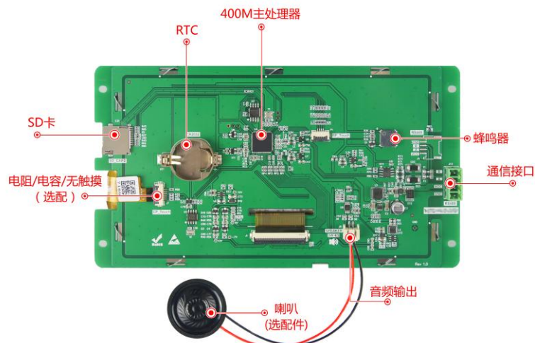
图 1-4 硬件配置图
