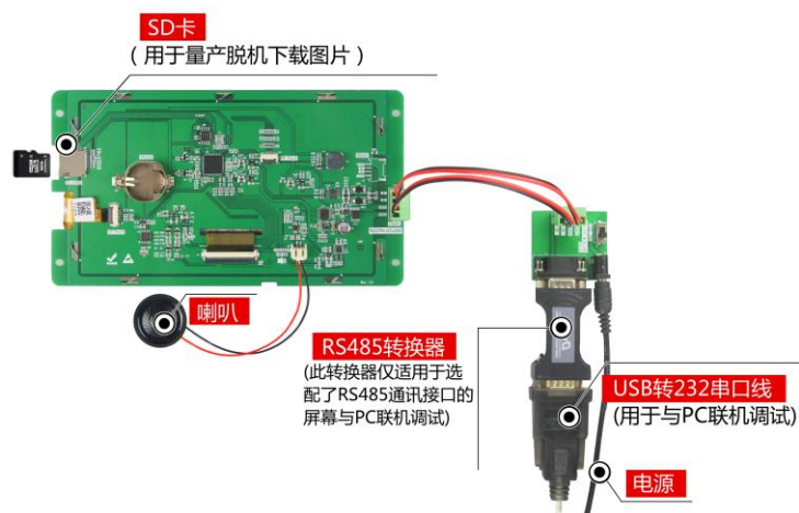
图 1-5 调试工具图
