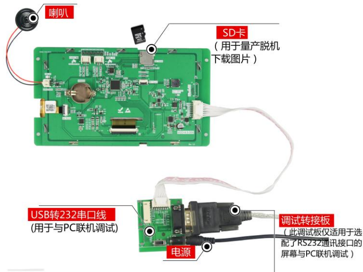
图 1-5 调试工具图
