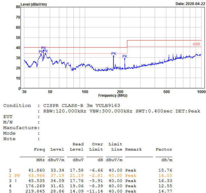
图 4-6 RE 测试垂直方向
