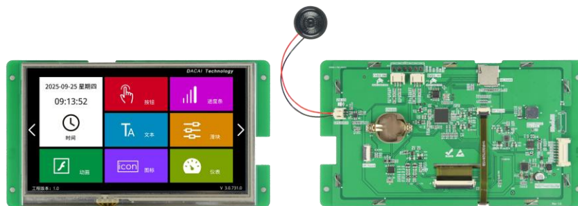
图 1-1 7.0 寸电阻触摸参考图
