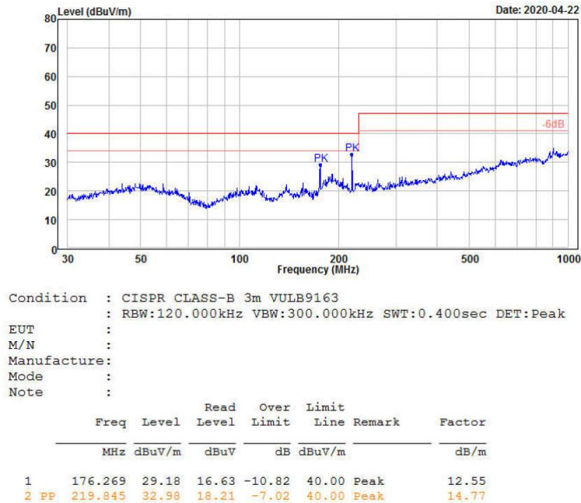
图 4-5 RE 测试水平方向
