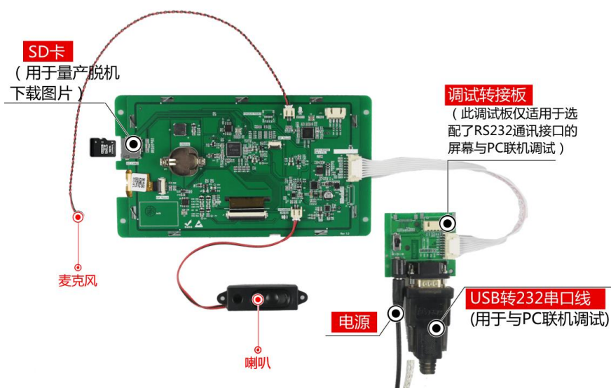
图 1-5 调试工具图
