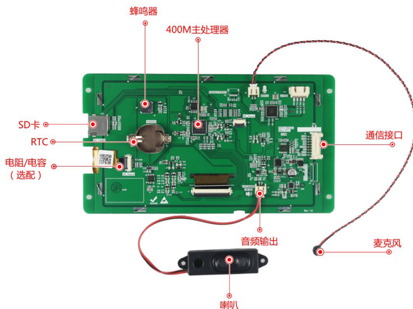
图 1-4 硬件配置图
