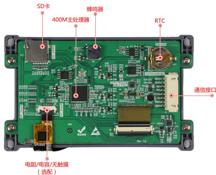
图 1-4 硬件配置图
