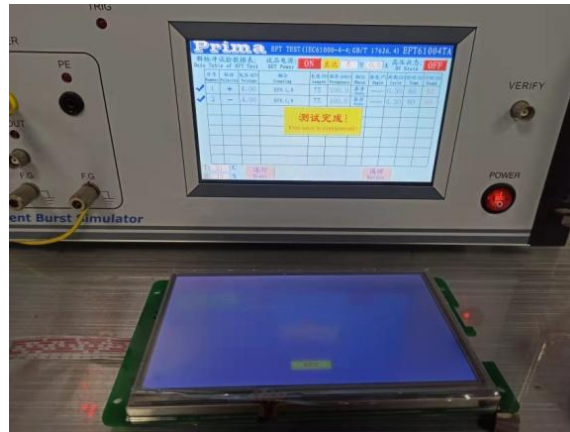
图 4-3 EFT 测试图
