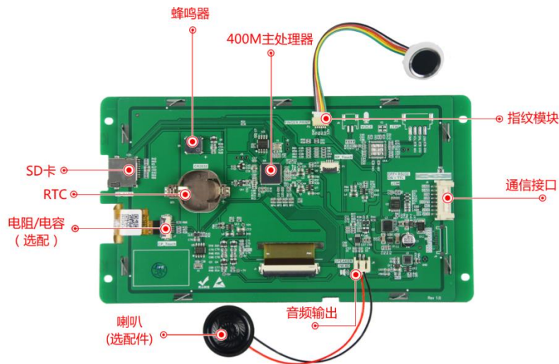
图 1-4 硬件配置图
